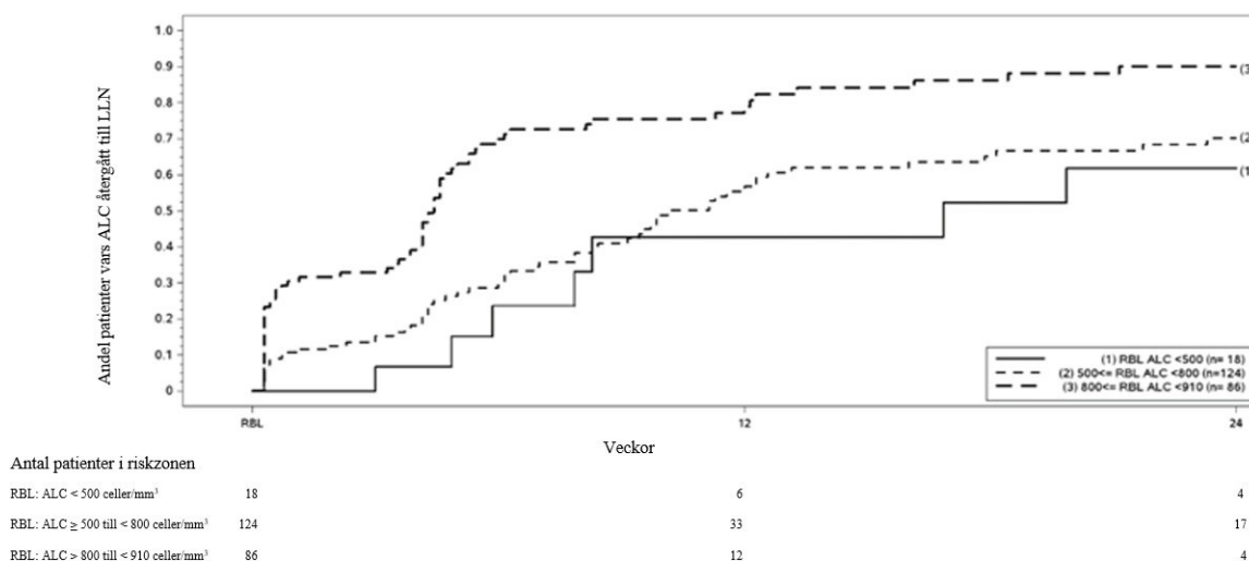
Figur 1: Kaplan-Meier-metod: andel patienter med återhämtning till \geq 910 \text{ celler/mm}^3 LLN från baslinjevärdet för återhämtning (RBL)
