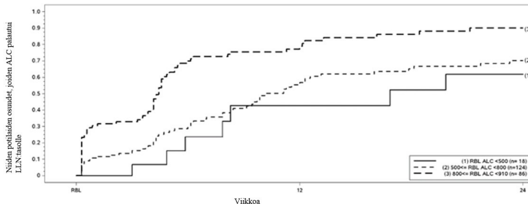
Kuva 1: Kaplan–Meierin menetelmällä arvioitujen niiden potilaiden osuudet, joiden absoluuttinen lymfosyttimäärä (ALC) palautui palautumisen lähtötilanteesta (RBL) normaaliarvojen alarajaan (LLN) ( \geq 910 solua/mm 3 )
